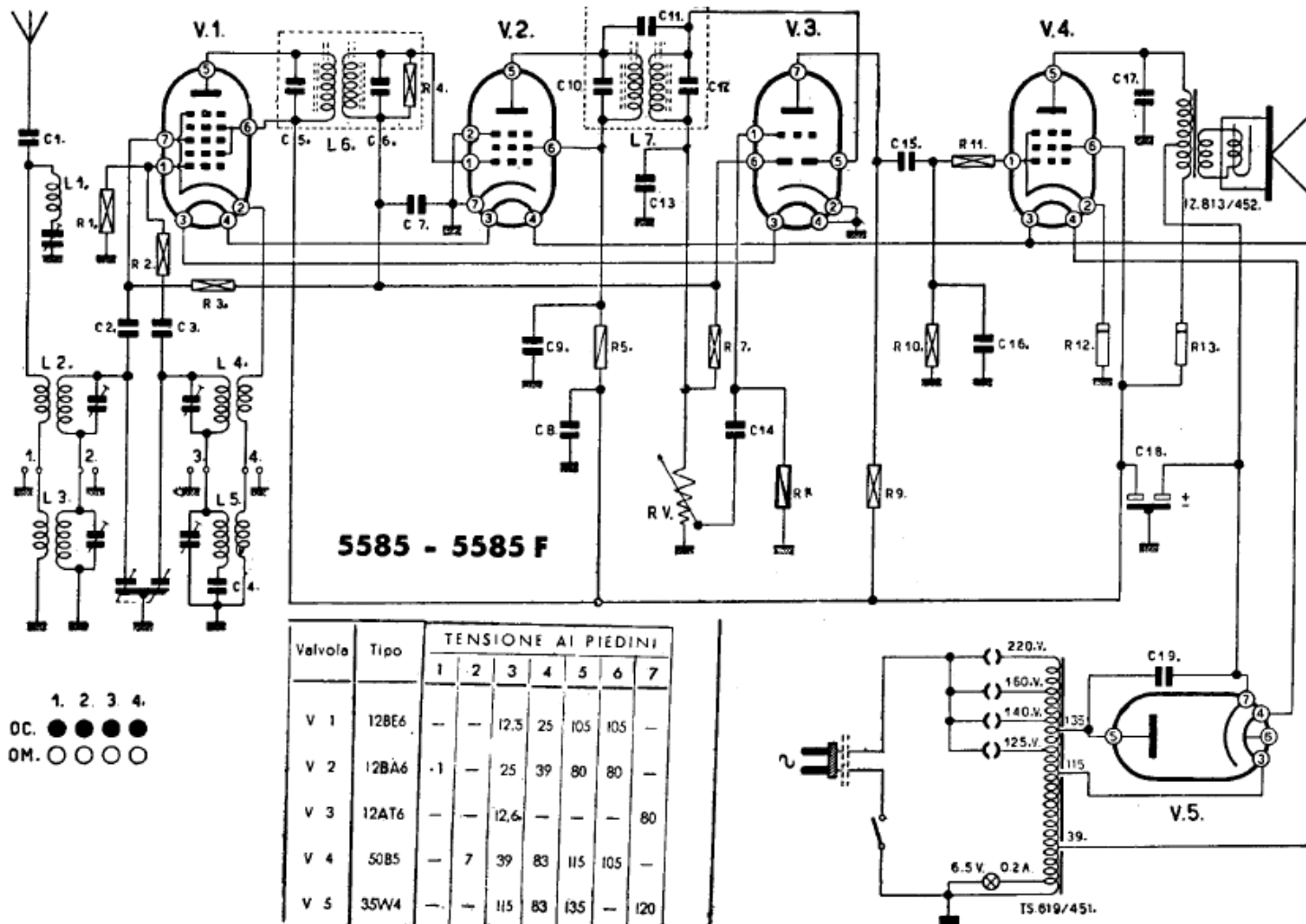
PHONOLA (S. A. FIMI) - Modd. 5585 e 5585 F. Onde medie e onde corte. Media frequenza a 468 kc/s. Lo schema è del mod. 5585; v. variante a parte per il mod. 5585 F. Potenza 2,3 watt.
